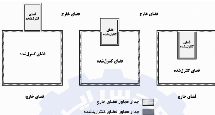
شکل 2- موقعیت جدارهای مجاور خارج و مجاور فضای کنترل نشده در پلان شماتیک سه نمونه ساختمان
